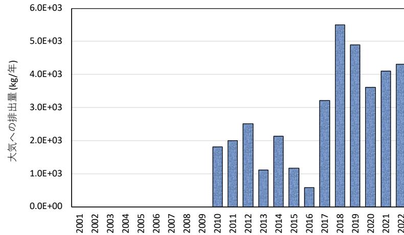
1-ブロモプロパン
