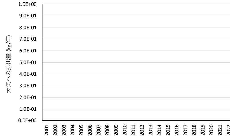
ヒドラジン
