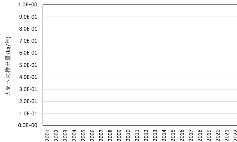
二硫化炭素
