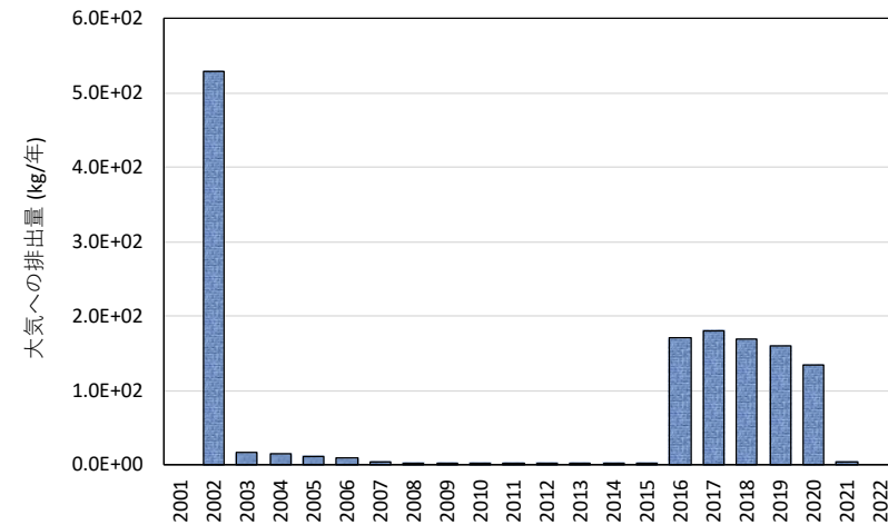
ヒドラジン
