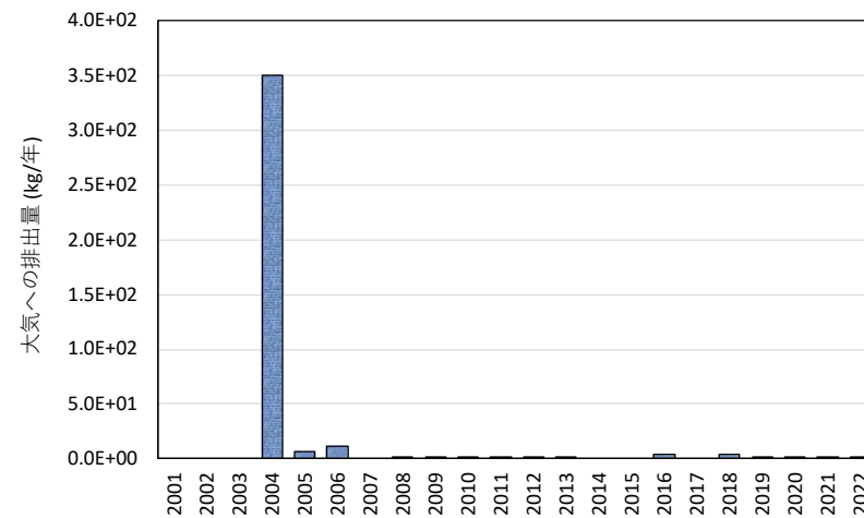
ヒドラジン
