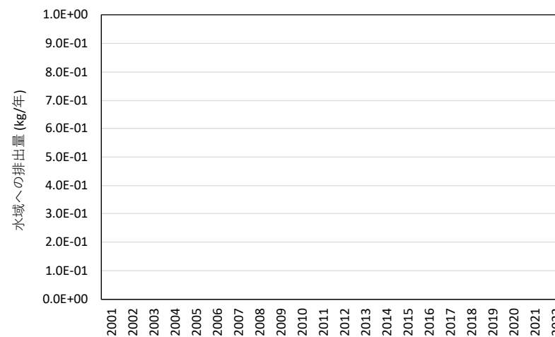
二硫化炭素
