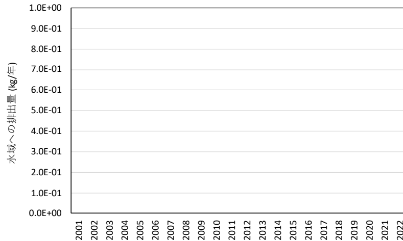
ピリジン
