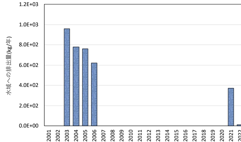
ヒドラジン
